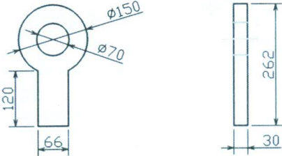
PÁT MỐC THÙNG (dùng thép tấm dày 30 mm)
